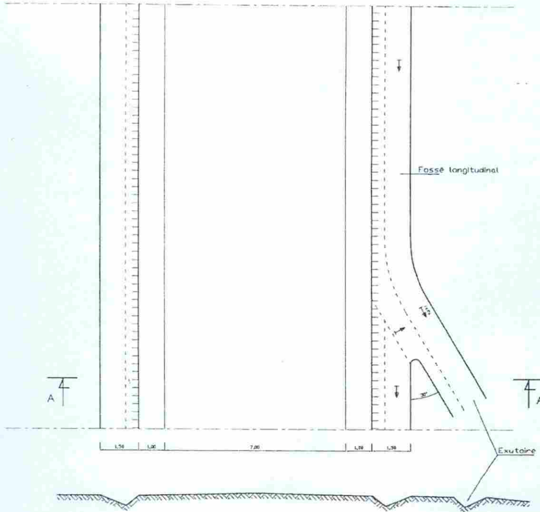
COUPE A-A
